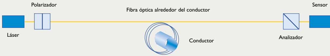
Esquema de medida de campos magnéticos utilizando una fibra óptica enrollada al conductor.
